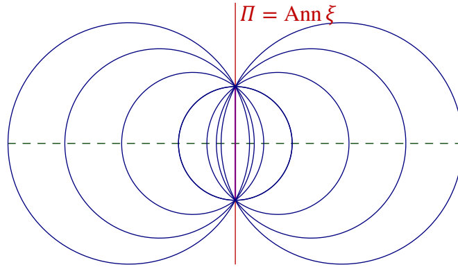
Рис. 23◊7. Пучок пересекающихся сфер.
