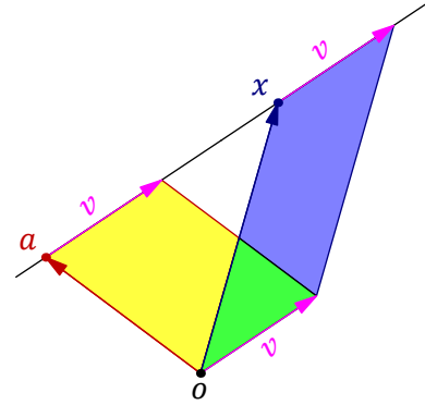
Рис. 1◊7. Уравнение прямой.
