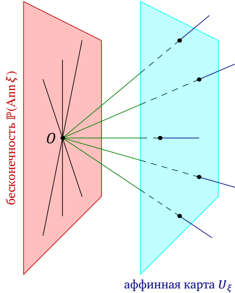
Рис. 17◊1. Проективный мир.
