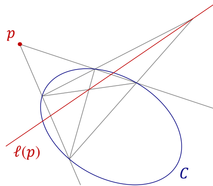
Рис. 18◊14. Построение поляр.
