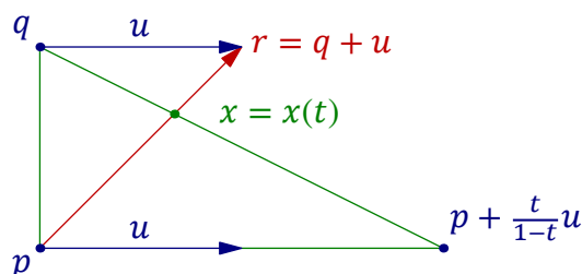
Рис. 13◊5. \overline{px} : \overline{xr} = t : (1-t) .
