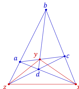
Рис. 18.1. Четырёхвершинник.
