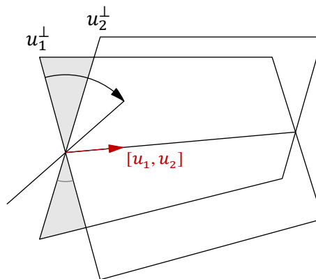
Рис. 12◊2. Поворот.
