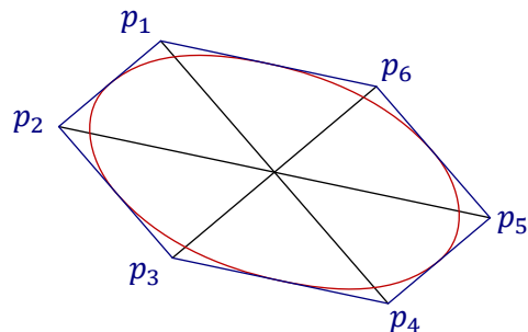
Рис. 19◊3. Описанный шестиугольник.
