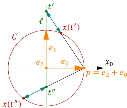
Рис. 17◊9. Параметризация окружности.
