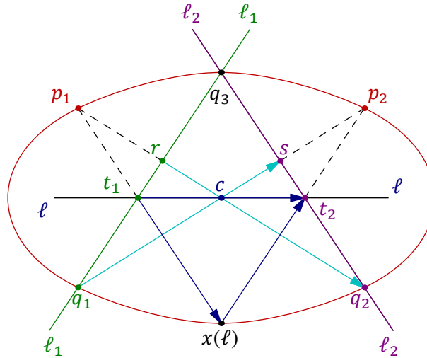
Рис. 18◊6. Трассировка коники линейкой.
