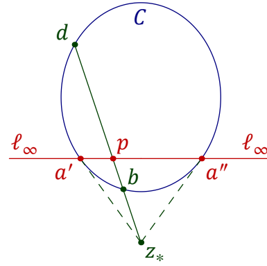
Рис. 21◊2. Центральная коника.
