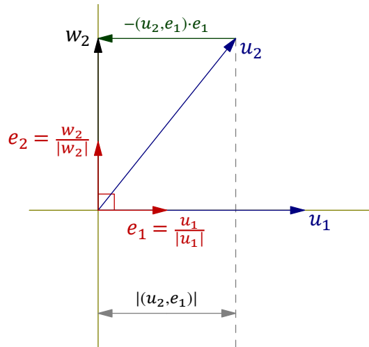
Рис. 11◊1. Второй шаг ортогонализации.
