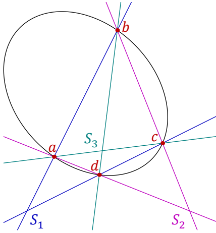
Рис. 20◊5. Простой пучок.
