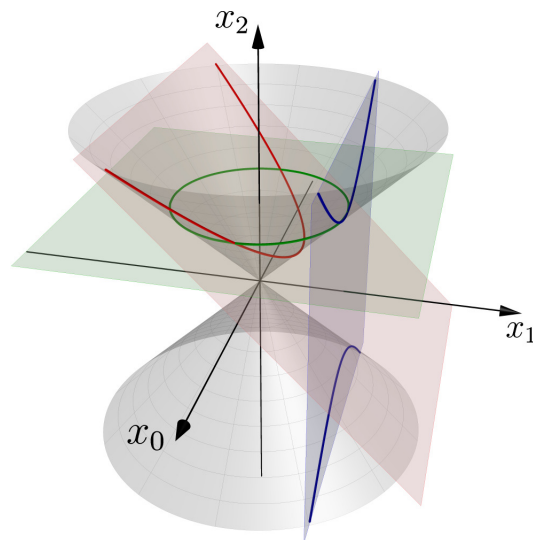
Рис. 17◊7. Аффинные изображения проективной коники.
