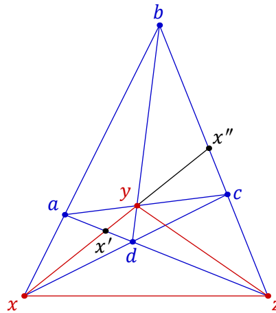
Рис. 18.10.
