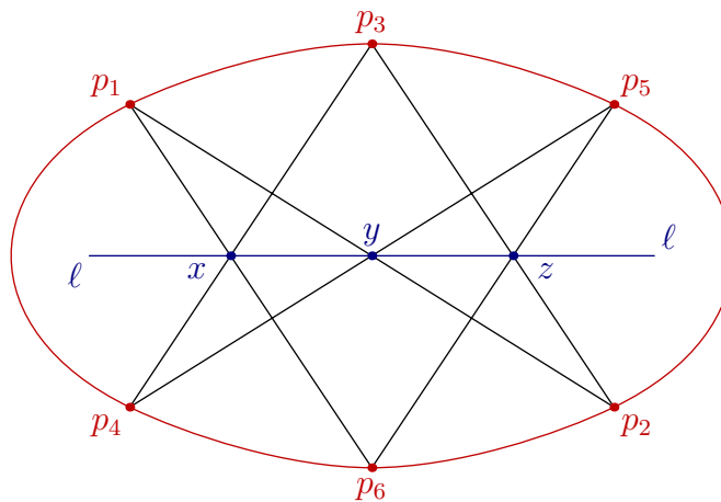
Рис. 18◊7. Гексограмма Паскаля.
