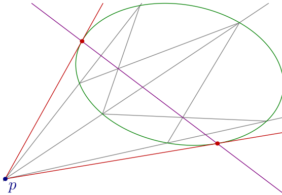
Рис. 18◊13. Построение касательных.
