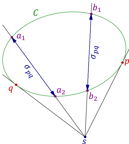
Рис. 18◊11. Инволюция на конике.
