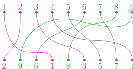
Рис. 8♦3. \operatorname{sgn}(2, 9, 6, 1, 8, 3, 5, 7, 4) = +1 (всего 18 пересечений).
