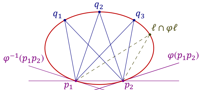
Рис. 18◊9. Неperспективная гомография \varphi : p_1^\times \rightarrow p_2^\times .
