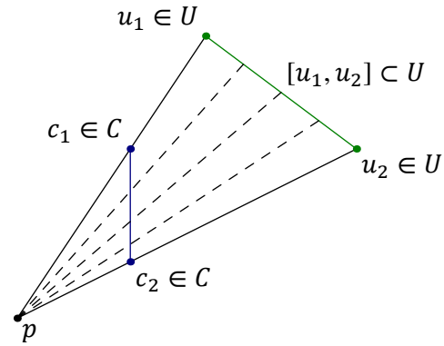
Рис. 13◊3. Выпуклость C .
