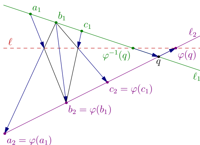
Рис. 18◊3. Перекрёстная ось.
