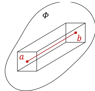
Рис. 13◊1. Выпуклость внутреннейности.
